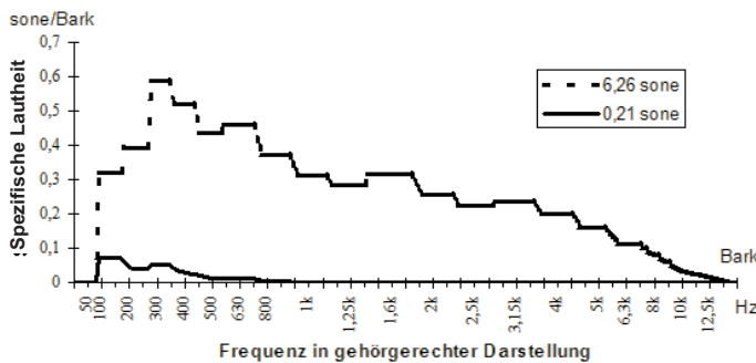
Bild 2 : Geräuschpegel an einem Schnittplatz (AVID) Verwendung eines offenen Racks - SAGA maxi plus
