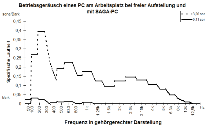
Bild 2 : Geräuschpegel an einer Workstation freistehender PC - PC in SAGA PC XL
